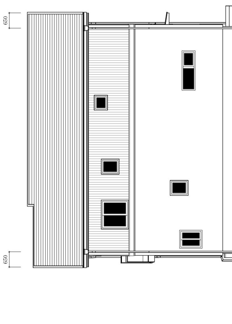
南側 立面図 S:1/100
